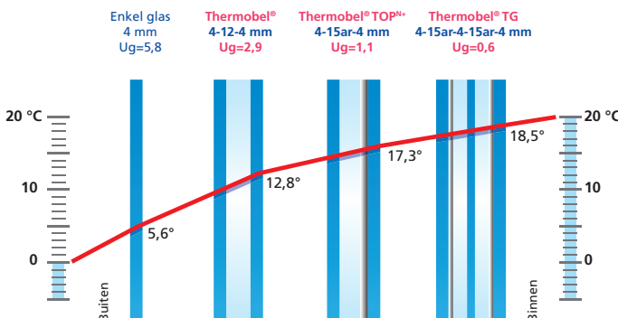
Temperatuurvariaties aan de binnenzijde van de beglazing in functie van de Ug-waarde.
